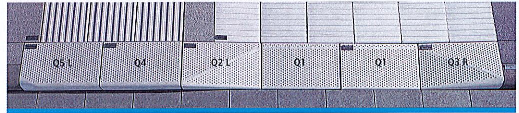
Getrennte Querungsstellen mit Bodenindikatoren Fußgängerüberwege mit F15 Verkehrsinsel
