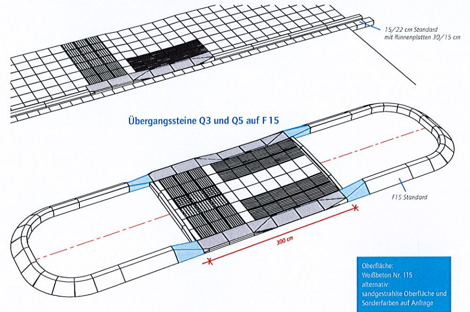
Getrennte Querungsstellen mit Bodenindikatoren Fußgängerüberwege mit F15 Verkehrsinsel
