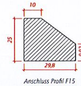
Anschluss Profil F15
