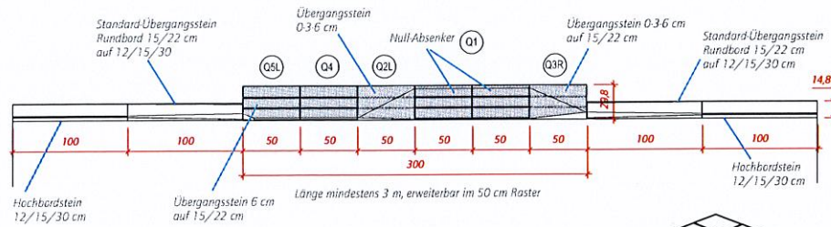
Draufsicht (Maßeinheiten in cm)
